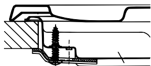
Монтаж крюка для опорных брусков H=20 мм
